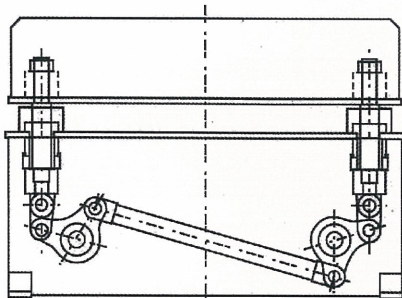
オートバランスシステム構造(特許)
